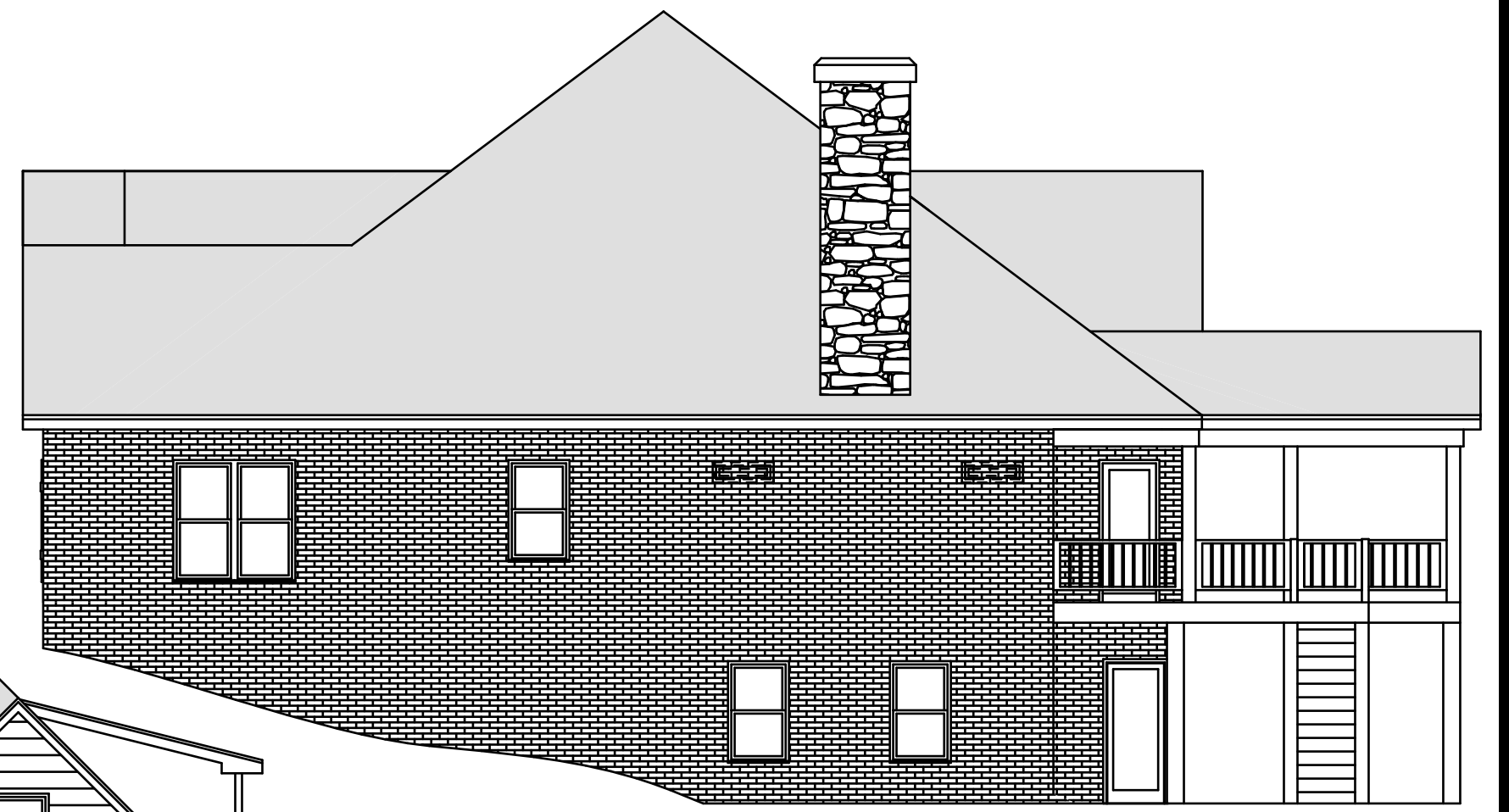
RIGHT ELEVATION
